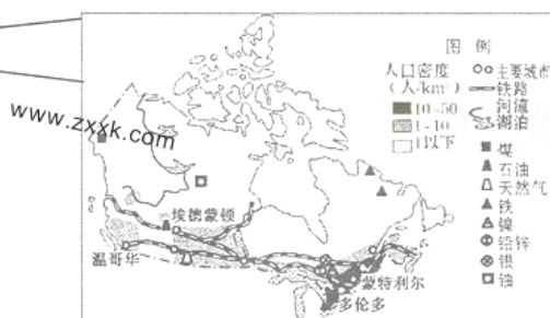
图2 加拿大矿产、人口分布
