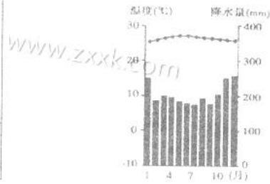
图2 新加坡气温曲线和降水柱状图
