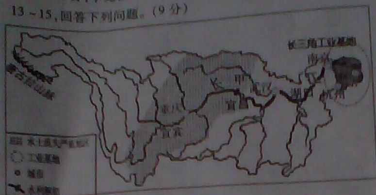
图13 长江流域图
